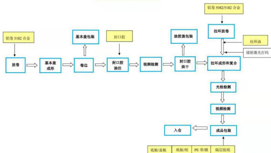
易拉盖工艺流程图
